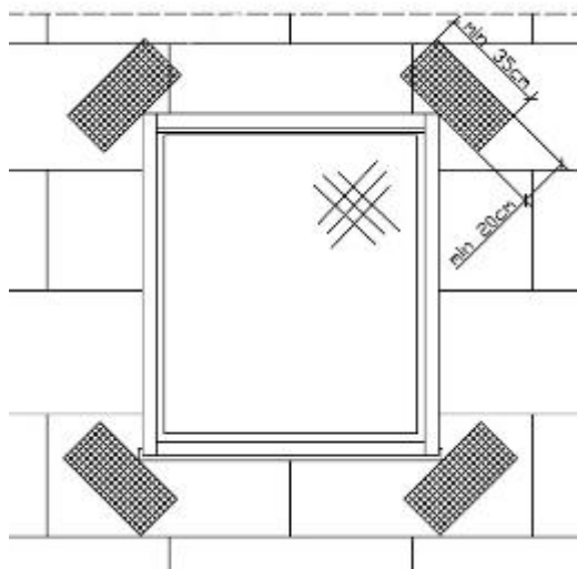
rys. 3. Wzmocnienie naroży otworów
